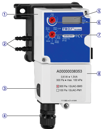
Universalregler XD4, Typ GUAC-SM3
