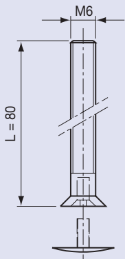
Zentralschraube mit Abdeckkappe für Typ DDQ F, DD F und DDRQ F
