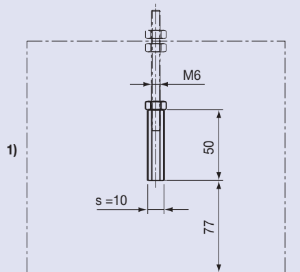
Gewinde-Rohr-Kupplung GRM6 für Typ DDQ F, DD F und DDRQ F
