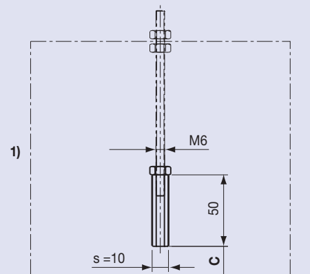
Gewinde-Rohr-Kupplung GRM6 für Typ DDQ K, DD K und DDRQ K
